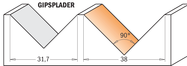
Tegning er 1:1
